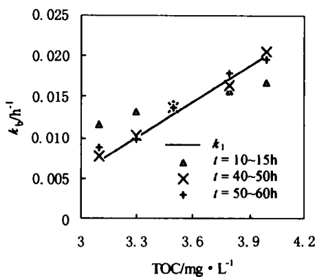
图6 衰减常数与 TOC 的关系
