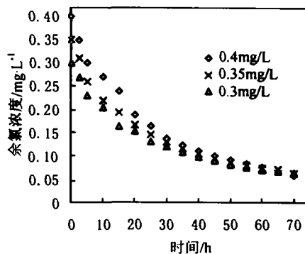
图 2 15°C, TOC = 3.5\text{mg}\cdot\text{L}^{-1} 时不同 c_0 对氯衰减的影响
