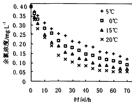
图 3 TOC = 3.5\text{mg}\cdot\text{L}^{-1} , c_0 = 0.4\text{mg}\cdot\text{L}^{-1} 时不同温度对氯衰减的影响
