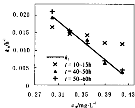
图7 衰减常数与 c_0 的关系
