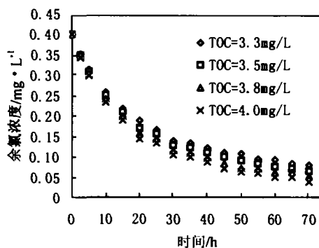
图 1 15°C, c_0 = 0.4\text{mg}\cdot\text{L}^{-1} 时不同 TOC 对氯衰减的影响
